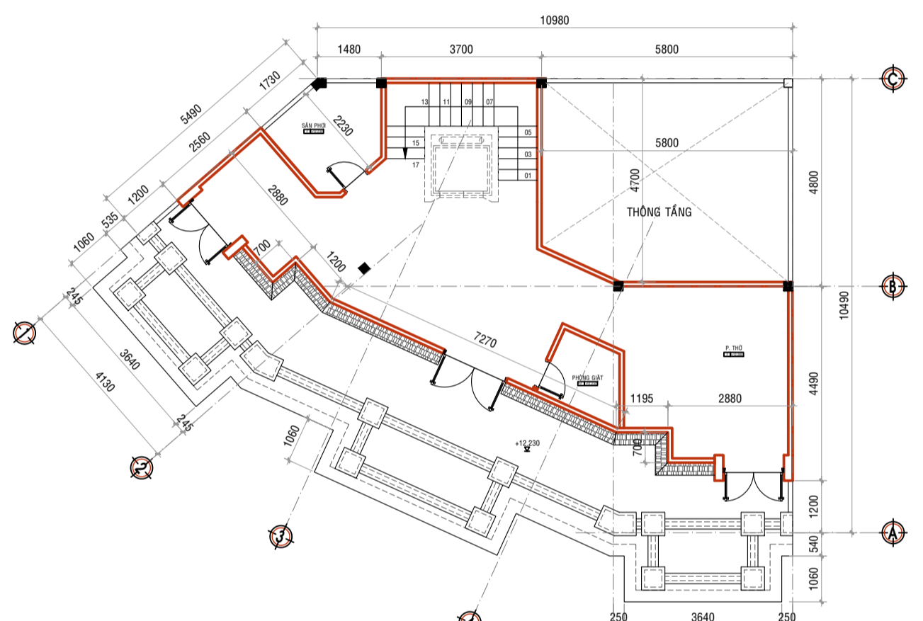
MẶT BẰNG TẦNG 4 TL: 1/100
