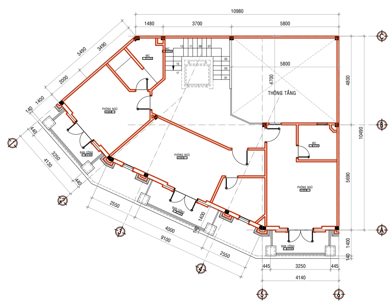
MẶT BẰNG TẦNG 2 TL: 1/100
