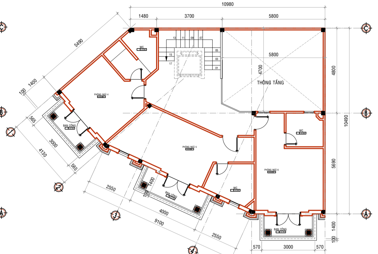
MẶT BẰNG TẦNG 3 TL: 1/100
