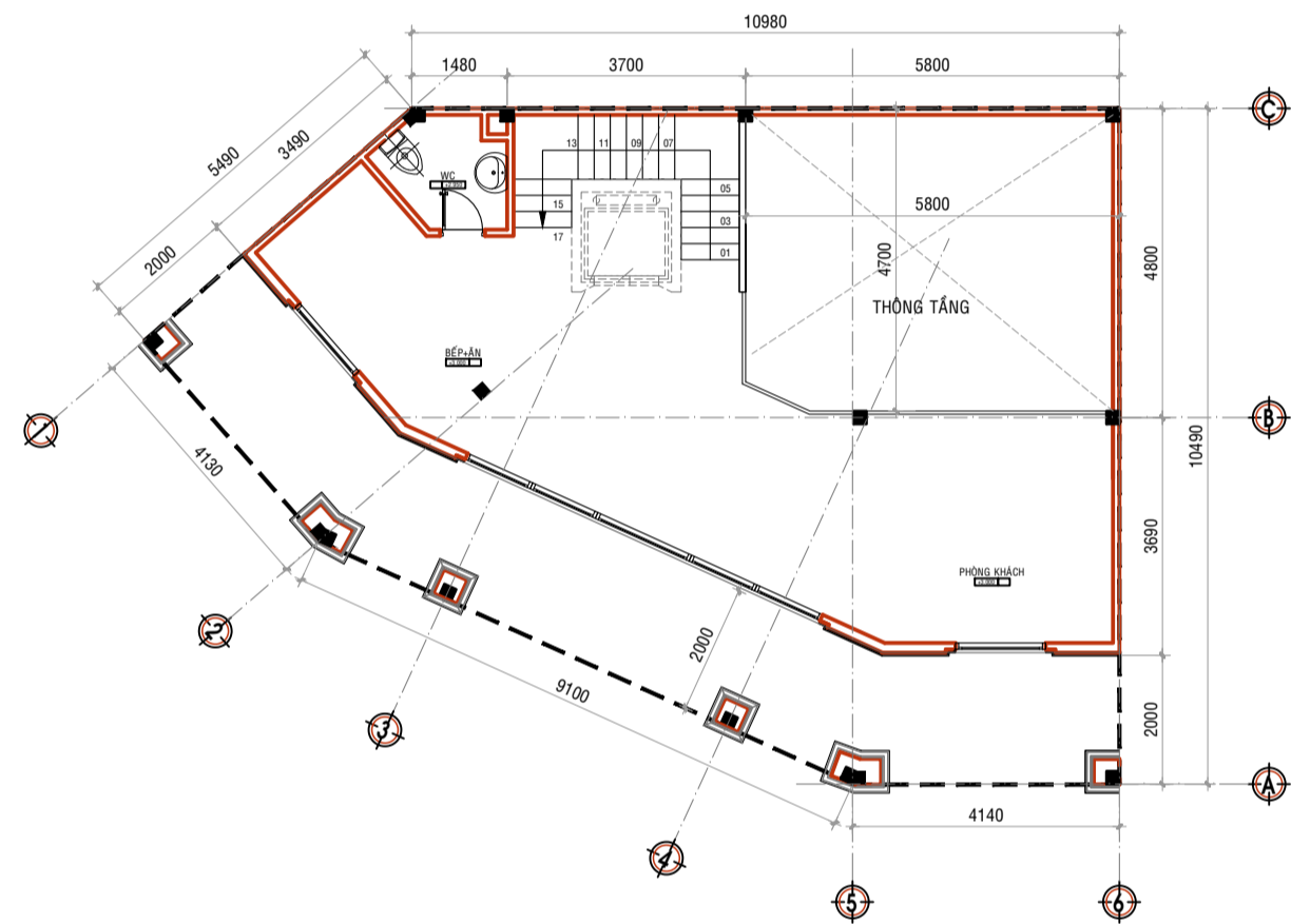
MẶT BẰNG LỬNG TL: 1/100
